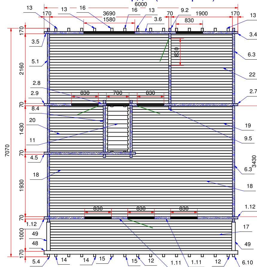
План мансарды (house plan)
