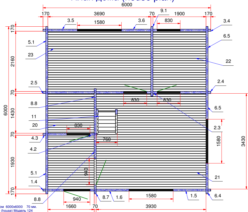
План дома (house plan)
