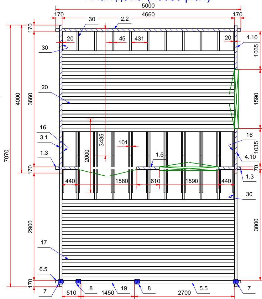
План дома (house plan)
