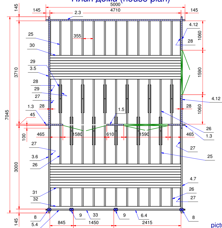
План дома (house plan)
