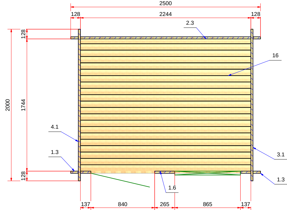
План дома (house plan)
