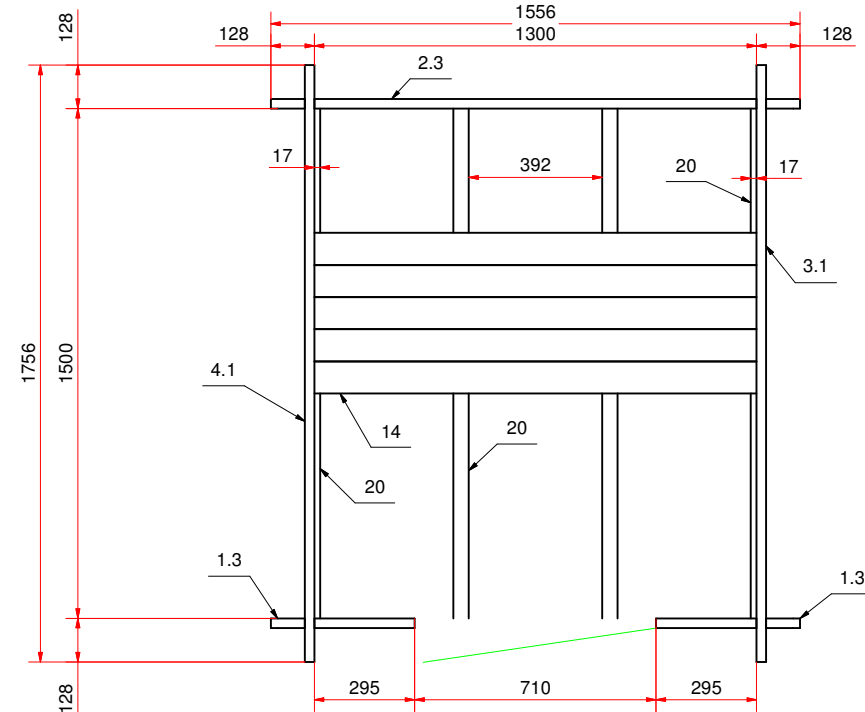
План дома (house plan)
