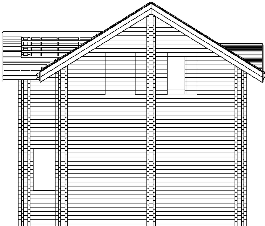
Фасад в осях 1 - 2
